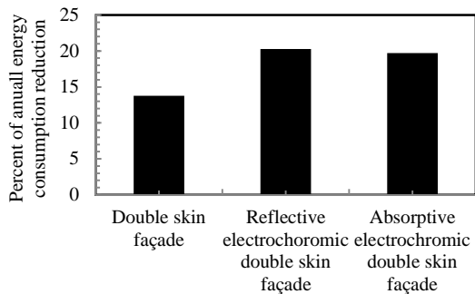
Fig. 6 The comparison of annual energy consumption of building شکل 6 مقایسه میزان مصرف انرژی سالانه ساختمان
