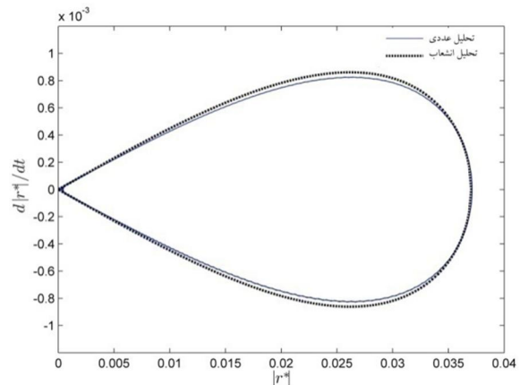
شکل 11 نمودار فاز یک روتور غیرخطی غیر میرا m^* = 0.3 , \alpha^* = 50 , \alpha_R^* = 50 , R^* = 0.25 , \omega_0^2 = 0.1 , \Omega^* = 5.1 , v = 0.2 , l^* = 0.1 , f = 0.2 , \mu^* = 0 , \mu_b^* = 0
