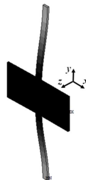
شکل 2 مد اول ارتعاش تشدیدگر مستطیلی میکرومکانیکی با دو تیر نگهدارنده قائم، مد شناور
