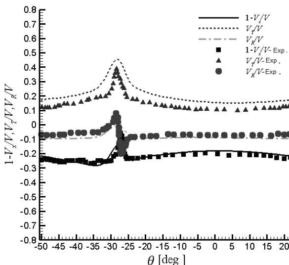
Fig. 8 مولفه های دنباله جریان در r/R = 0.7, x/D = 0.1 و J = 1.25
