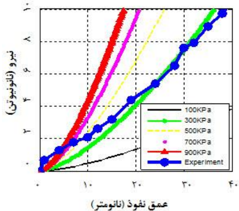
شکل ۱۲) نمایش مدل تماسی جی‌کآر و نتایج تجربی در نمودار نیرو-عمق نفوذ
