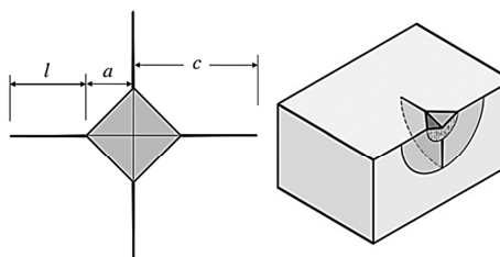
الف - اثر سوزن ویکرز و طول ترک
