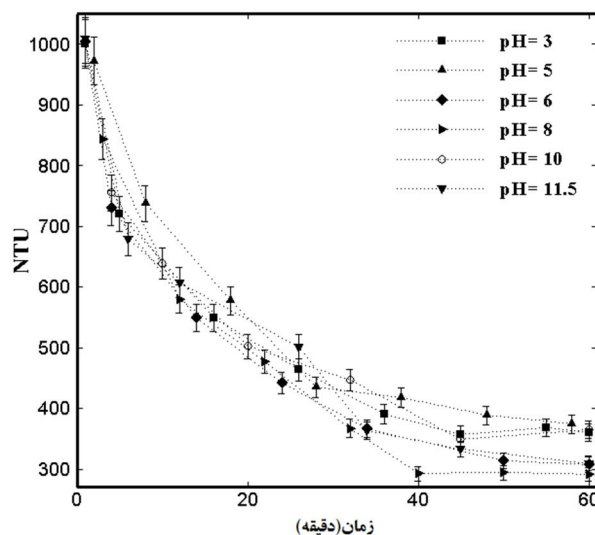
شکل 11 تغییر کدورت مخلوط میکروذرات و نانوذرات بر حسب زمان و در کوتاه مدت با غلظت نانوذرات و میکروذرات \varphi_{\text{micro}} = 1.098 \times 10^{-4} و \varphi_{\text{nano}} = 5.0 \times 10^{-4}
