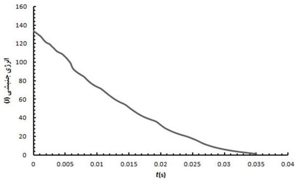
شکل 30 نمودار تغییرات انرژی جنبشی چکش در جاذب S 3
