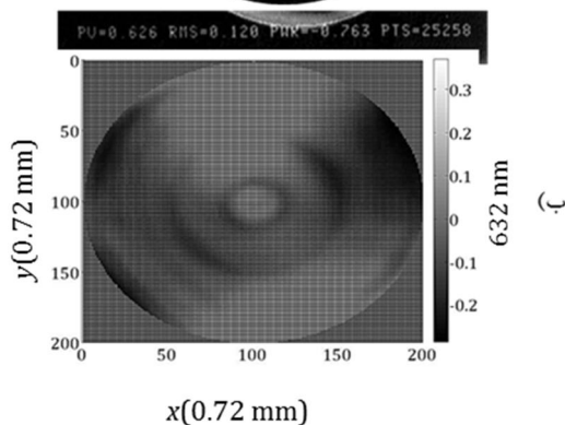
شکل 11 (الف) فرایج‌های سطح بعد از پرداخت (ب) ماتریس سطح بعد از پرداخت (با بزرگنمایی \frac{1}{0.72} )
