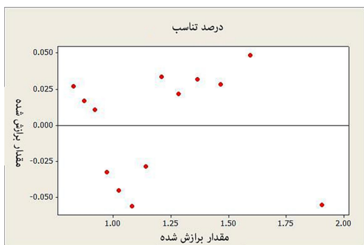
شکل ۶ مقادیر مانده‌ها در برابر مقادیر برازش شده برای خروجی
