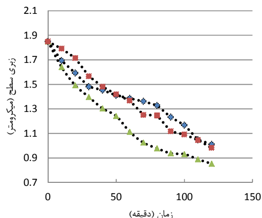
شکل ۵ اثر تغییرات زبری سطح در زمان
