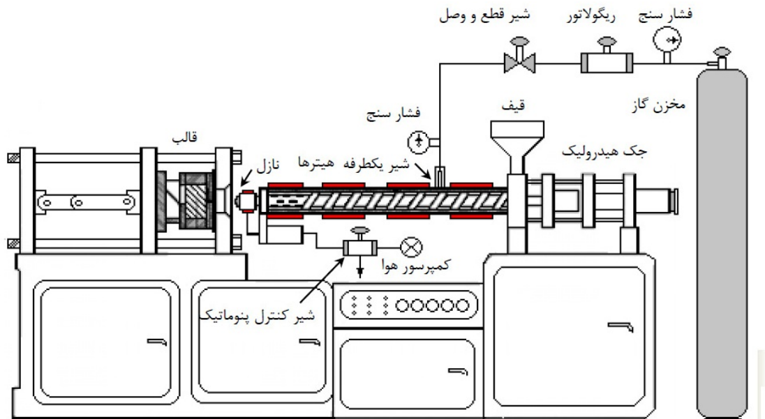
شکل ۲ شمای کلی دستگاه تزریق معمولی که با نصب تجهیزات لازم، توانایی تولید قطعات فوم ریزسلولی را دارد
