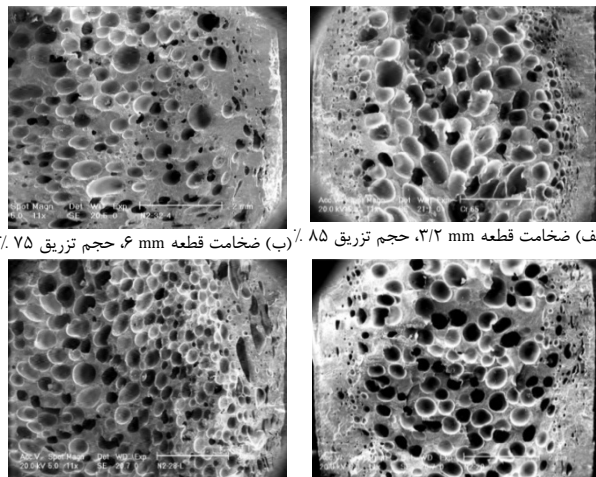
شکل ۷ تصاویر SEM از مقاطع نمونه‌ها در ضخامت‌های مختلف (پهنای دریچه ثانویه ۷ mm)
