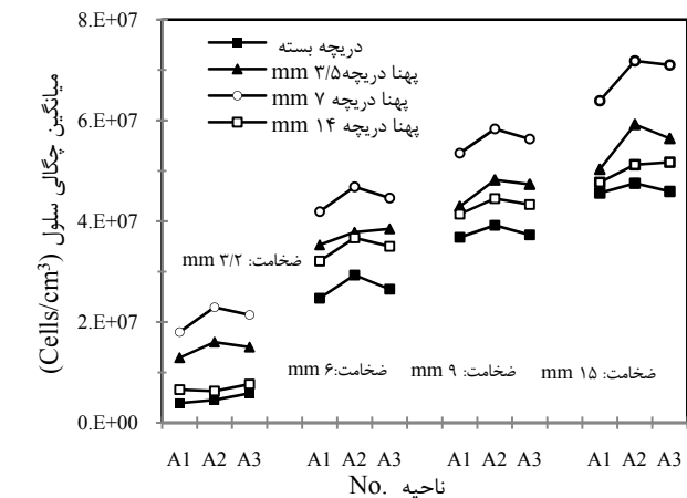
شکل ۹ اثر دریچه ثانویه بر چگالی سلول در سه ناحیه انتخاب شده
