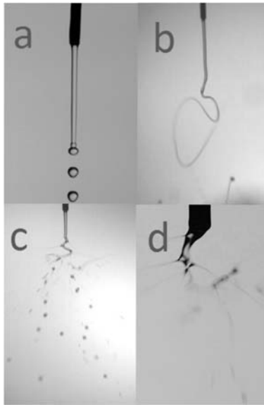
Fig. 16 The other modes, Flowrate= 250 ml/h, (a): Simple jet, Voltage= 3.92kV, (2): Oscillating simple jet, Voltage= 6.01kV, (c) Ramified jet, Voltage= 9.66kV, Random spray, Voltage= 12.81kV. شکل 16 سایر حالت‌های پاشش، دبی سیال 250 ml/h، ولتاژ (a): جت ساده، ولتاژ اعمالی 3.92kV، (b): جت ساده نوسانی، ولتاژ اعمالی 6.01kV، (c): جت منشعب، ولتاژ اعمالی 9.66kV، (d): پاشش تصادفی، ولتاژ اعمالی 12.81kV.
