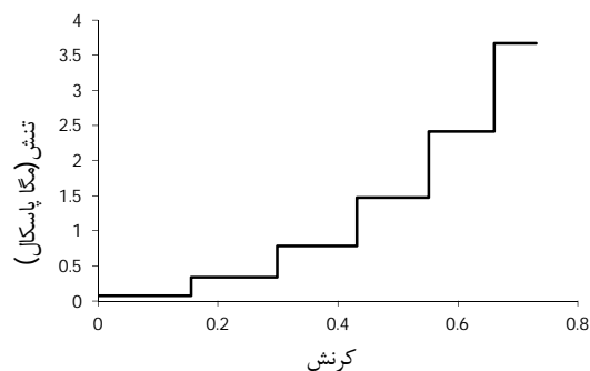
شکل 5 نمودار تنش - کرنش سازه لانه زنبوری مدرج
