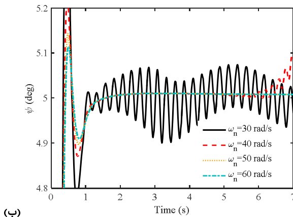
نمودار ۴) (الف) زاویه سمت در اثر دستور اعمالی ۵ درجه بدون اعمال ضرایب دینامیکی و در فرکانس‌های طبیعی مختلف عملگر، (ب) نمودار بزرگ‌نمایی شده
