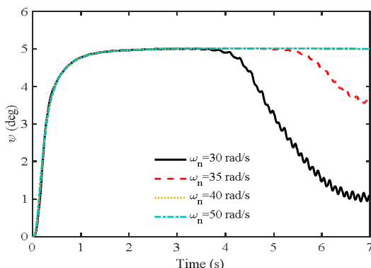
نمودار (۷) زاویه سمت در اثر دستور اعمالی ۵ درجه با اعمال ضرایب دینامیکی و در فرکانس‌های طبیعی مختلف عملگر
