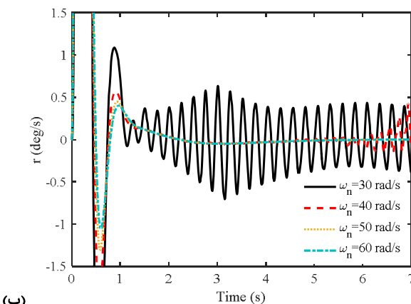
نمودار ۵) (الف) نرخ زاویه سمت در اثر دستور اعمالی ۵ درجه بدون اعمال ضرایب دینامیکی و در فرکانس‌های طبیعی مختلف عملگر، (ب) نمودار بزرگ‌نمایی شده
