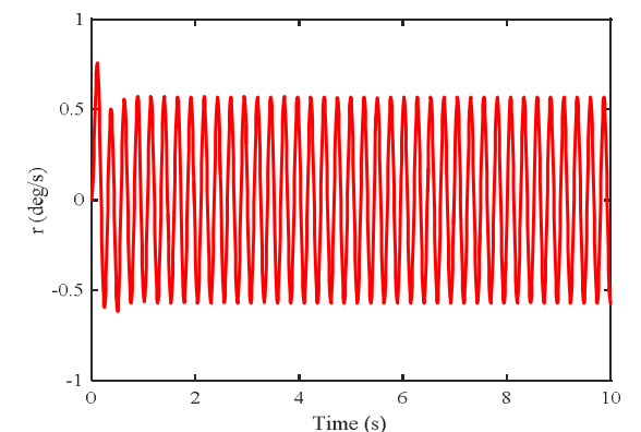
نمودار ۱۵) تغییرات نرخ زاویه سمت در اثر اعمال ورودی سینوسی با فرکانس ۳/۹ هرتز به دینامیک سیستم با اعمال ضرایب دینامیکی C_{N\dot{\beta}} و C_{Y\dot{\beta}} , C_{Y\dot{r}} , C_{N\dot{r}}
