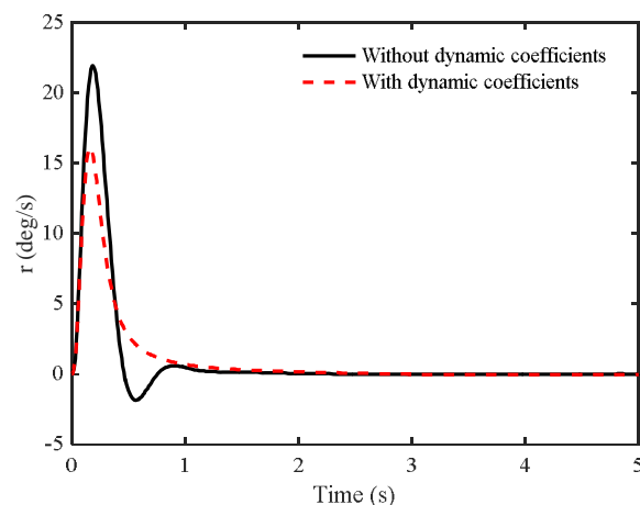
نمودار ۲) تغییرات نرخ زاویه سمت در اثر دستور اعمالی ۵ درجه در دو حالت اعمال ضرایب دینامیکی و چشم‌پوشی از ضرایب دینامیکی
