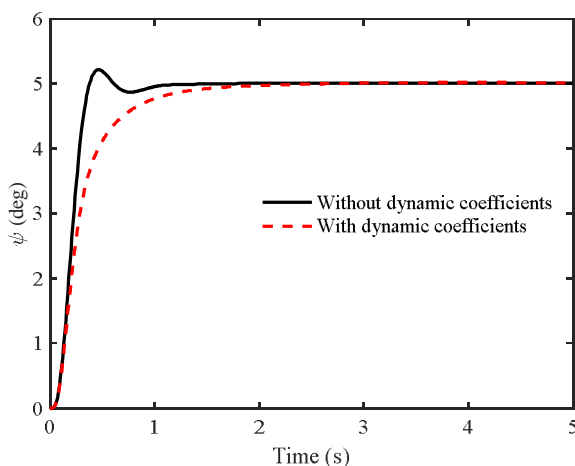
نمودار ۱) تغییرات زاویه سمت در اثر دستور اعمالی ۵ درجه در دو حالت اعمال ضرایب دینامیکی و چشم‌پوشی از ضرایب دینامیکی
