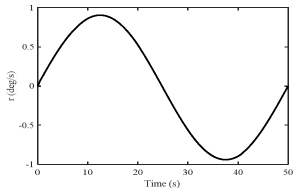
نمودار ۱۴) تغییرات نرخ زاویه سمت در اثر اعمال ورودی سینوسی با فرکانس ۰/۲ هرتز به دینامیک سیستم با اعمال ضرایب دینامیکی C_{N\dot{\beta}} و C_{Y\dot{\beta}} , C_{Y\dot{r}} , C_{N\dot{r}}
