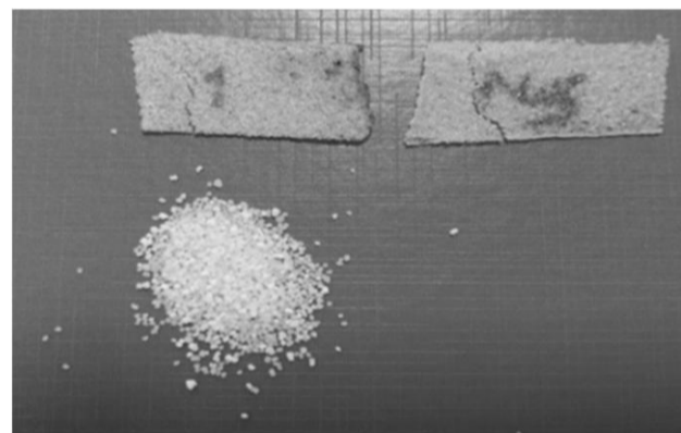
شکل 4 نمونه‌های شماره 1 و 5 سینتر شده توسط لیزر از پودر پلی پروپایلین
