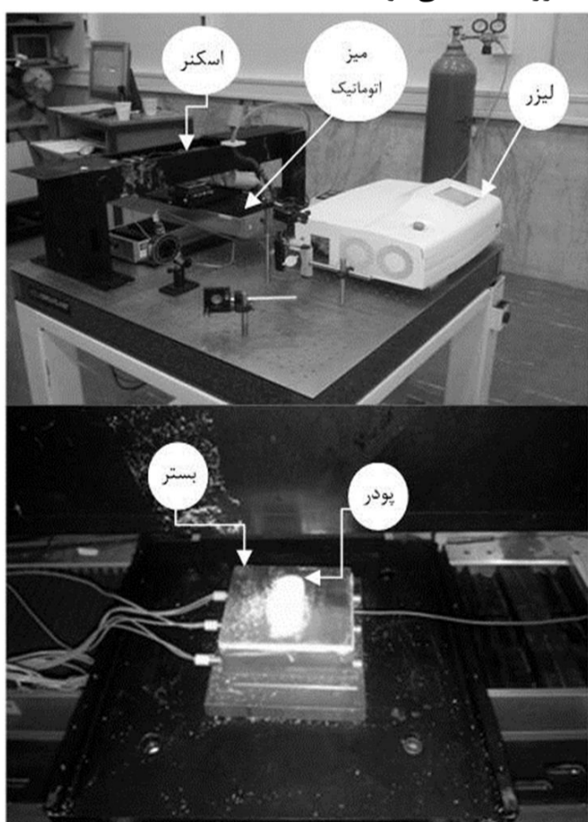
شکل 5 دستگاه ساخته شده برای سینترینگ لیزری
