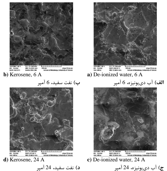
Fig. 9 Investigating surface cracks by SEM images with 500 X magnification for the 12.8 \mu s pulse on time شکل 9 بررسی ترک‌های سطحی به کمک تصاویر میکروسکوپ الکترونی با بزرگنمایی 500 برابر برای زمان روشنی پالس 12.8 میکروثانیه
