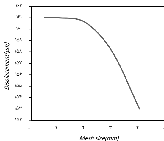
نمودار ۱) نمودار حساسیت به سائز مش در تست کشش
