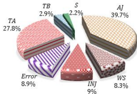
(ش) میزان تاثیر پارامترها بر نرخ برش (ارتفاع برش 90mm)
