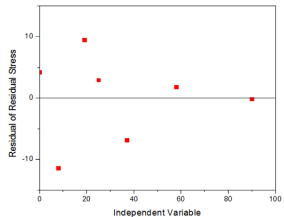
نمودار ۷) توزیع باقیمانده تنش‌های پسماند محوری در سطح خارجی لوله با استفاده از تابع چندجمله‌ای درون‌یاب درجه ۴
