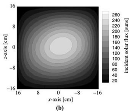
شکل ۵) توزیع شار خورشیدی ناشی از هلیوستات ۴۷ روی یک صفحه ۳۰×۳۰ سانتی‌متری واقع در مرکز کانونی متمرکزکننده سهموی؛ الف) نتایج اندازه‌گیری شده [29] ، ب) نتایج شبیه‌سازی شده
