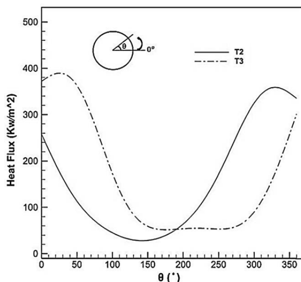
نمودار ۳) توزیع شار تابشی روی لوله‌های ۲ و ۳ در حالت راکتور مکعبی منعکس‌کننده
