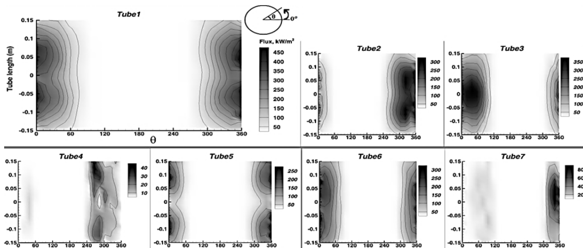
شکل ۸) شار تابشی ایجادشده روی لوله‌های داخل راکتور مکعبی کاملاً جاذب
