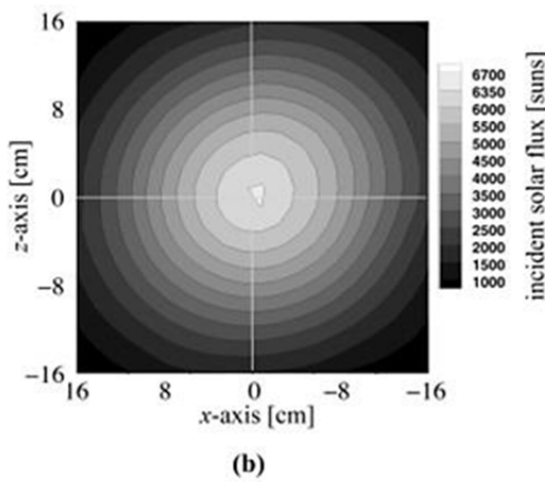
شکل ۶) توزیع شار خورشیدی حاصل از ۳۶ عدد از هلیوستات‌ها روی یک صفحه ۳۰×۳۰ سانتی‌متری واقع در مرکز کانونی متمرکزکننده سهموی؛ الف) نتایج اندازه‌گیری شده [30] ، ب) نتایج شبیه‌سازی شده
