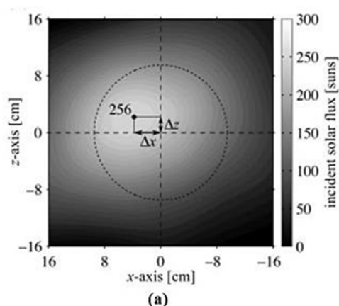
شکل ۵) توزیع شار خورشیدی ناشی از هلیوستات ۴۷ روی یک صفحه ۳۰×۳۰ سانتی‌متری واقع در مرکز کانونی متمرکزکننده سهموی؛ الف) نتایج اندازه‌گیری شده [29] ، ب) نتایج شبیه‌سازی شده
