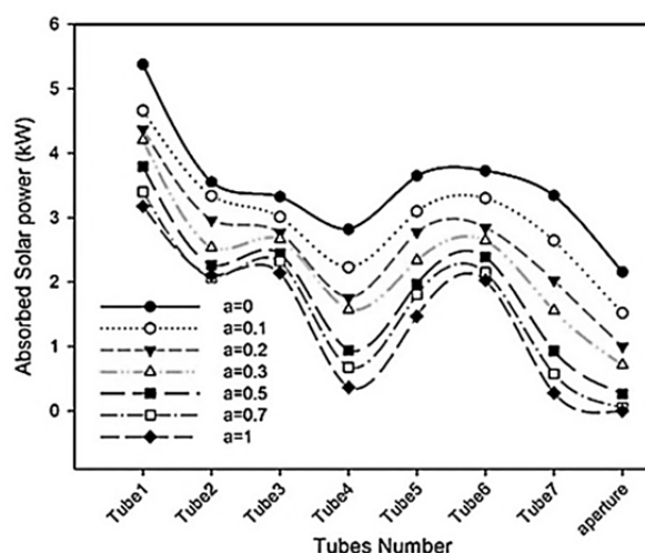
نمودار ۱) توان جذب‌شده توسط لوله‌های گرافیتی و توان بازتابش‌شده از روزنه در ضرایب جذب مختلف دیواره‌های راکتور
