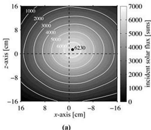
شکل ۶) توزیع شار خورشیدی حاصل از ۳۶ عدد از هلیوستات‌ها روی یک صفحه ۳۰×۳۰ سانتی‌متری واقع در مرکز کانونی متمرکزکننده سهموی؛ الف) نتایج اندازه‌گیری شده [30] ، ب) نتایج شبیه‌سازی شده
