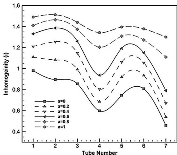
نمودار ۲) ضریب یکنواختی تابشی لوله‌های گرافیتی در ضرایب جذب مختلف دیواره‌های راکتور
