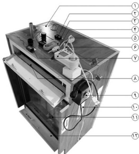
شکل ۳) مدول ساخته‌شده از پوسته هموستاتیک برای صحت‌سنجی پیشنهادها؛ (۱) فضای داخلی، (۲) ترمومتر، (۳) بادسنج، (۴) کلید گرم‌کننده، (۵) انرژی‌متر، (۶) لوله متصل به آبگرمکن خورشیدی، (۷) لوله تراوا، (۸) دریچه تیپ A (ارتباط‌دهنده محیط با فضای هموستاتیک)، (۹) دیمر، (۱۰) فضای هموستاتیک، (۱۱) لایه شیشه‌ای، (۱۲) دریچه تیپ A
