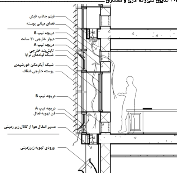
شکل ۴) برش دیواره هوشمند هموستاتیک از محل میان دو پنجره
