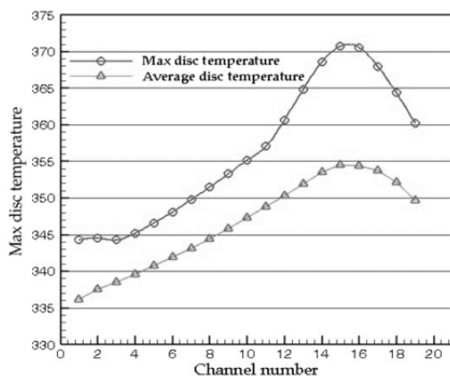
نمودار ۳) ماکزیمم و میانگین دمای دیسک‌ها
