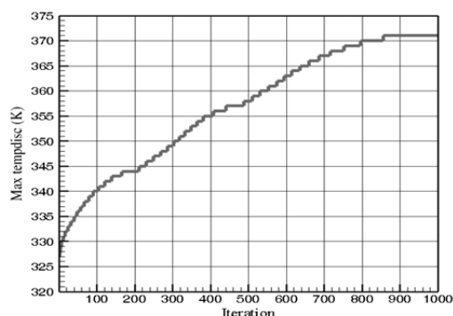
نمودار ۴) همگرایی دمای ماکزیمم دیسک‌ها
