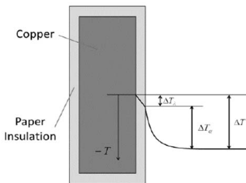
شکل ۳) گرادیان دما در داخل دیسک
