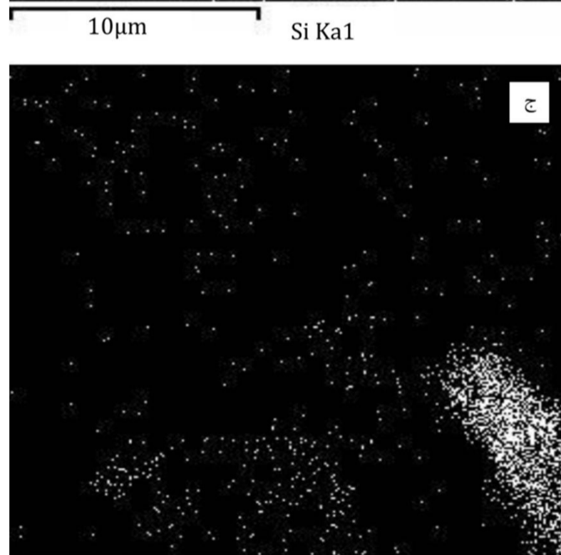
شکل 3 ریزنگارهای SEM گرفته شده همراه با EDX از ترکیبات پلی پروپیلن پر شده با گرافن و نانورس:
