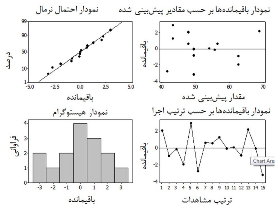
شکل 6 نمودارهای مربوط به باقیمانده‌ها
