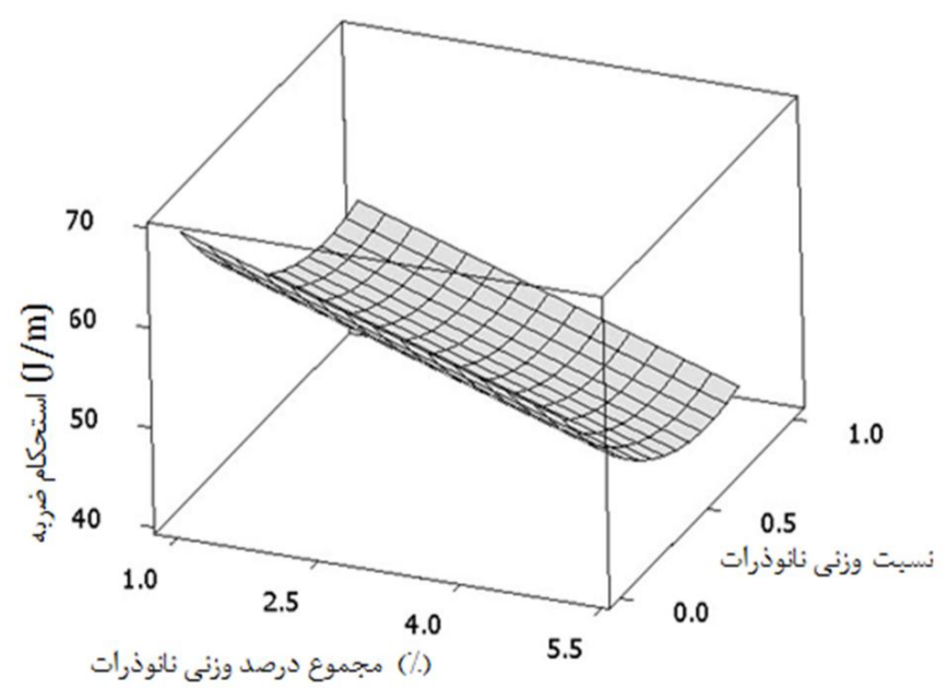
شکل 7 رویه پاسخ استحکام ضربه، مقدار ثابت: درصد وزنی PP-MA
