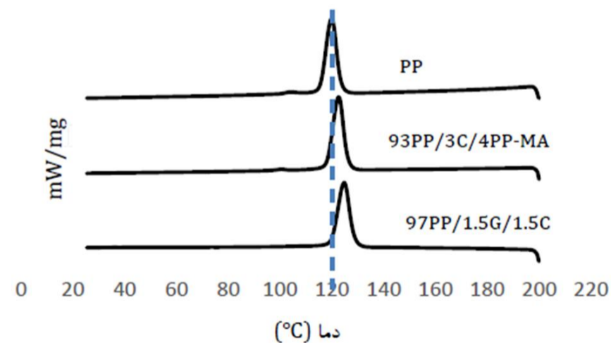
شکل 5 دمانگاشت DSC در فرآیند سرمایش برای پلی پروپیلن خالص و نمونه‌های 93PP/3C/4PP-MA و 97PP/1.5G/1.5C
