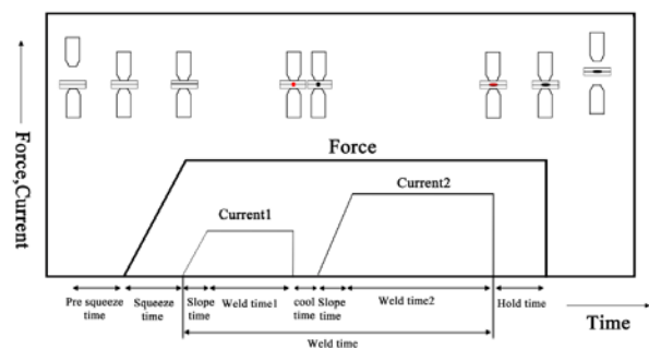
شکل ۱) چرخه جوشکاری مقاومتی نقطه‌ای و پارامترهای مؤثر در این فرآیند
