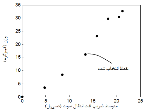
شکل ۸ نمایش جبهه پرتو نقطه انتخاب شده براساس روش تاپسیس برای پنل پنج‌لایه
