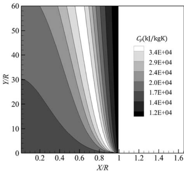
Fig. 21 Calculated contour of special heat capacity at constant pressure for carbon dioxide, \Delta T=3 , p=8\text{MPa} , T_{\text{avg}}=308.25 , D=0.3\text{mm} شکل 21 کانتور به‌دست‌آمده از ظرفیت گرمایی ویژه در فشار ثابت دی‌اکسید کربن، \Delta T=3 ، p=8\text{MPa} ، T_{\text{avg}}=308.25 ، D=0.3\text{mm}
