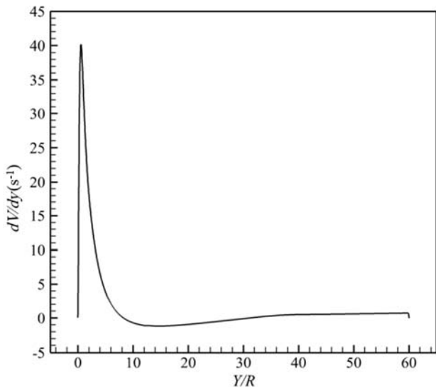
Fig. 20 Vertical velocity gradient at R=0.05\text{mm} for \Delta T=2 , p=8\text{MPa} , T_{\text{avg}}=307.75 , D=0.3\text{mm} شکل 20 گرادیان سرعت عمودی در R=0.05\text{mm} برای، \Delta T=2 ، p=8\text{MPa} ، T_{\text{avg}}=307.75 ، D=0.3\text{mm}
