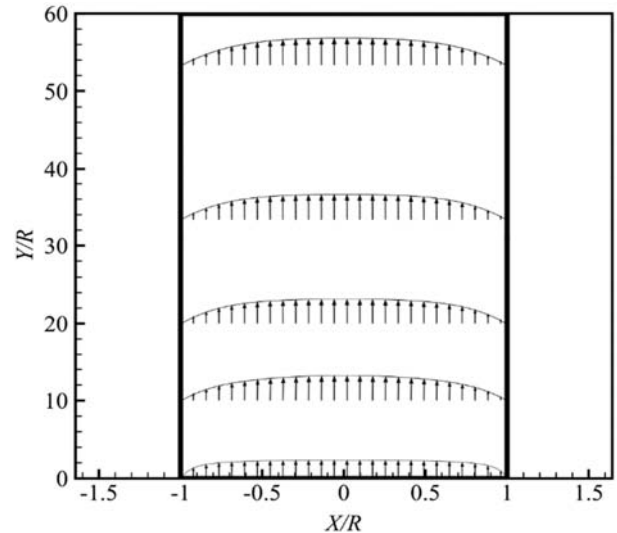
Fig. 19 Velocity profiles obtained from current study in various sections, \Delta T=1 , p=8\text{MPa} , T_{\text{avg}}=307.5 , D=0.2\text{mm} شکل 19 پروفیل‌های سرعت حاصل از تحقیق حاضر در مقاطع مختلف لوله، \Delta T=1 ، p=8\text{MPa} ، T_{\text{avg}}=307.5 ، D=0.2\text{mm}
