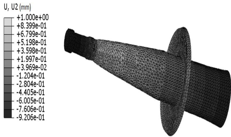
شکل 6 تحلیل نهایی ابزار ارتعاشی به منظور محاسبه فرکانس تشدید
