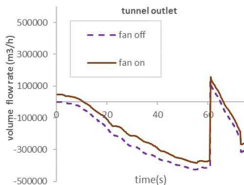
نمودار ۶) مقایسه تغییرات دبی هوا نسبت به زمان روی صفحه‌ای در انتهای تونل در حالت‌های فن روشن و فن خاموش
