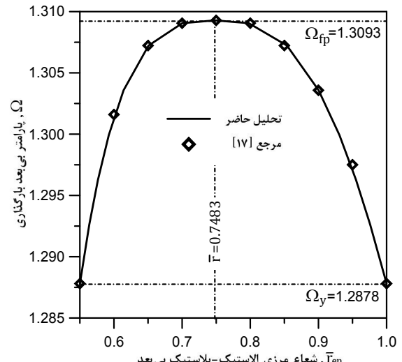
شکل ۷ پیشروی ناحیه پلاستیک هم‌زمان از شعاع داخلی و خارجی به‌ازای (a/b)=0/55 ، n_E=1/3826 ، (n_p=n_\sigma=0) و \Omega_{fp}=1/3093
