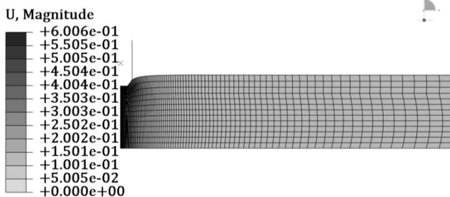
شکل 8 میزان فرورفتگی نشان داده شده در نرم‌افزار آباکوس (نمونه 1)
