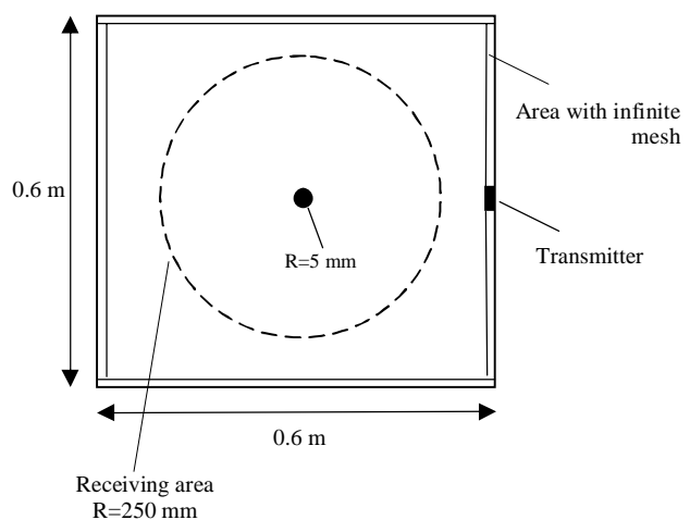
Fig. 4 Geometry of sample in scattering from a through-thickness hole شکل 4 هندسه قطعه در آزمون بررسی پراکندگی از سوراخ استوانه‌ای راه‌به‌در
