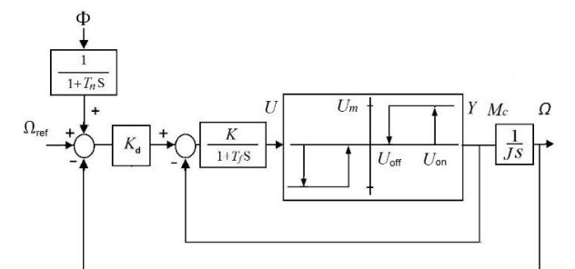
Fig. 1 Satellite attitude stabilization/tumbling with PWWF modulator شکل 1 پایدارسازی وضعیت/ دوران‌دهی ماهواره با مدولاتور پهنا و فرکانس پالس
