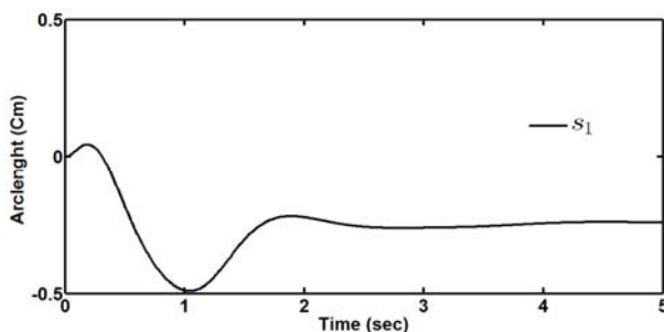
Fig 8. Trajectory of arc length parameter s_1
