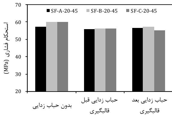
شکل ۱۶ میزان استحکام فشاری در ۹ فوم تولیدی به ۹ روش مختلف با ۶۰٪ حجمی میکروبالن و قالبگیری پس از ۴۵ دقیقه هم‌زدن نهایی
