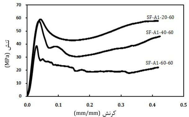
شکل ۱۲ نمودار تنش-کرنش برای سه فوم با درصد حجمی متفاوت میکروبالن
