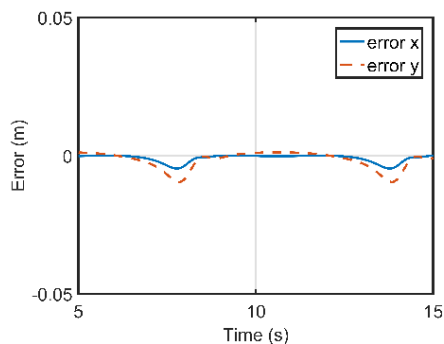
نمودار ۱۳) خطای مکانی ربات دوکابلی با کنترلر و در نظرگرفتن دست بیمار بعد از ثانیه پنجم
