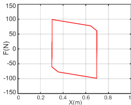
نمودار ۶) ناحیه کاری دینامیکی ربات تک‌کابل
