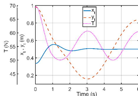
نمودار ۹) پارامترهای کنترلی ربات تک‌کابلی برای حرکت روی مسیر خطی
