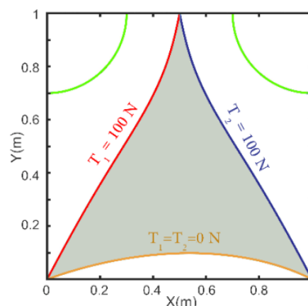
نمودار ۵) ناحیه کاری استاتیکی ربات دوکابل در روش حل تحلیلی
