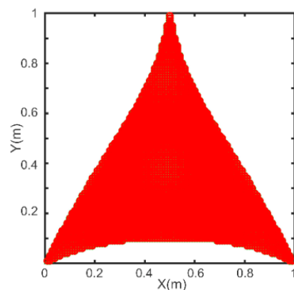
نمودار ۴) ناحیه کاری استاتیکی ربات دوکابل در روش حل عددی
