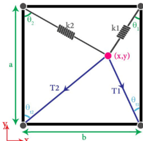
شکل ۷) شماتیک ربات دوکابل
