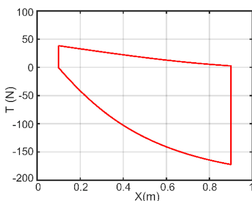
نمودار ۷) ناحیه کاری دینامیکی ربات دوکابل
