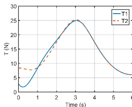
نمودار ۱۱) پارامترهای کنترلی ربات دوکابلی با کنترلر CTM
