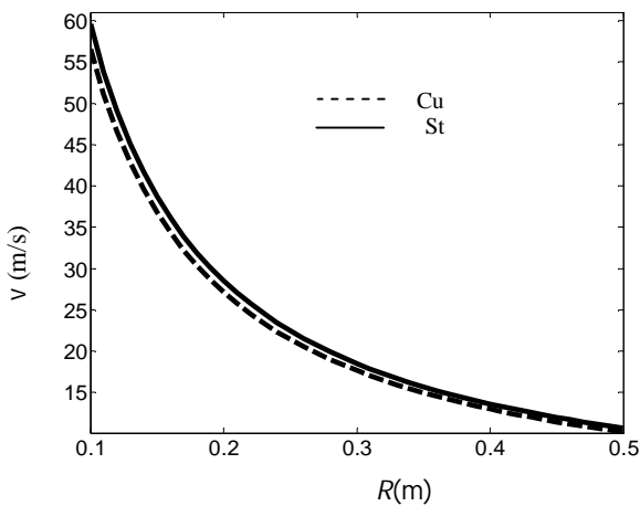
شکل 7 سرعت مركز ورق برحسب محل استقرار ماده‌ي منفجره در زمان كاويتاسيون
