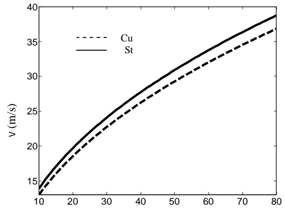
شکل 4 سرعت مركز ورق برحسب جرم ماده‌ي منفجره در زمان كاويتاسيون
