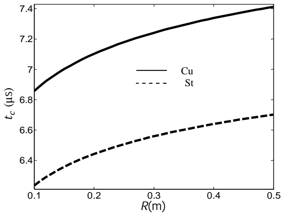
شکل 6 زمان كاويتاسيون برحسب محل استقرار ماده‌ي منفجره
