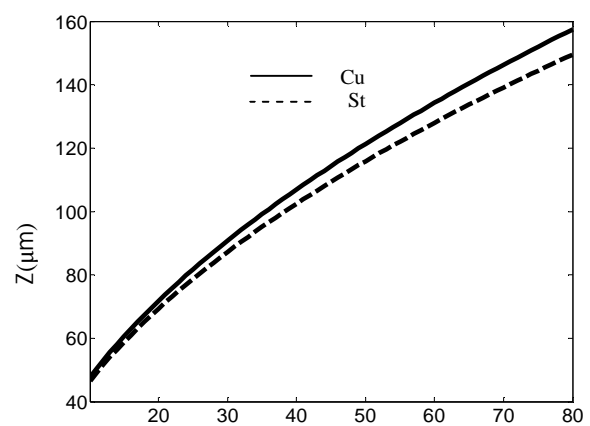
شکل 5 جابجايي مركز ورق برحسب جرم ماده‌ي منفجره در زمان كاويتاسيون
