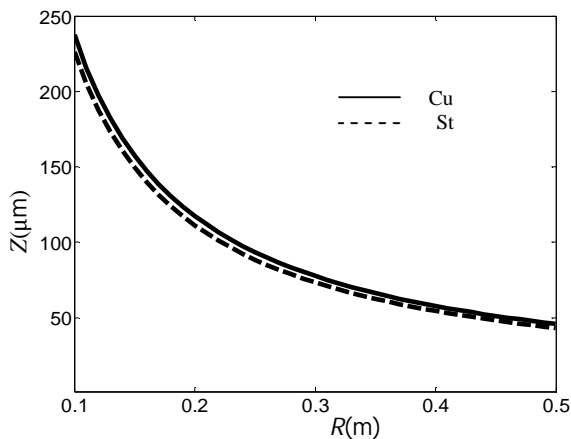
شکل 8 جابجايي مركز ورق برحسب محل استقرار ماده‌ي منفجره در زمان كاويتاسيون
