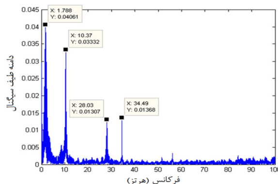
شکل ۱۵ جابه جایی FFT (ضربه ۵۰ ولت، میراگر فعال)
