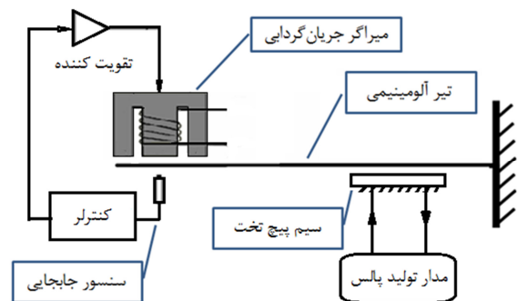
شکل ۵ چیدمان اجزاء آزمایش
