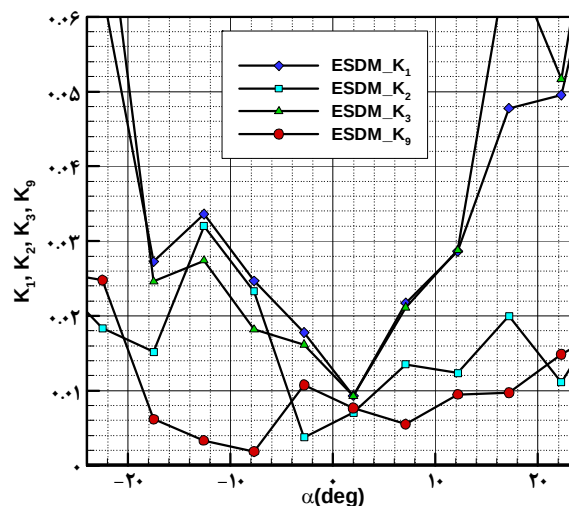
نمودار (۱۲) مقایسه مقدار خطای ESDM ضرایب K_1 و K_2 و K_3 و K_9 حسگر سه‌سوراخه با زاویه انحراف جریان
