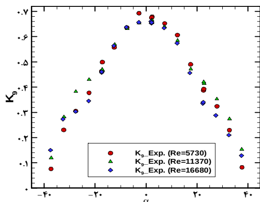
نمودار ۱۱) نمودار تغییرات ضریب K_9 حسگر سه‌سوراخه با زاویه انحراف جریان در روش تجربی
