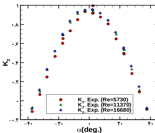
نمودار ۱۰) تغییر ضریب K_2 در روش تجربی با زاویه انحراف جریان
