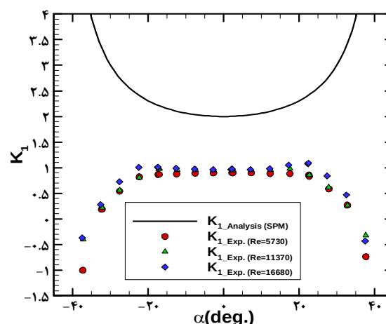
نمودار ۹) تغییر ضریب K_1 در روش تحلیلی و تجربی با تغییر زاویه انحراف جریان
