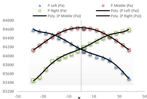
نمودار ۲) نمونه نمودار تغییرات فشار حسگر سه‌سوراخه با زاویه انحراف جریان در سرعت ۳۰ متر بر ثانیه
