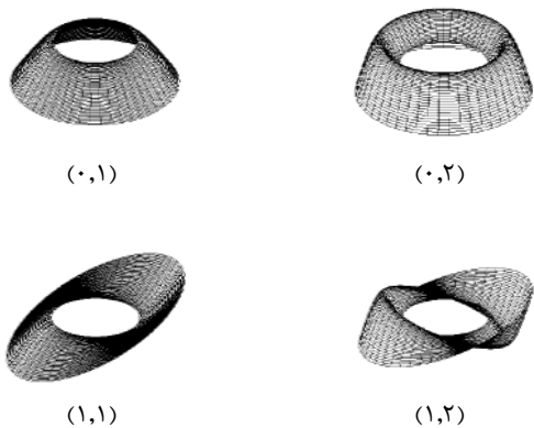
شکل ۴ شکل مدهای (m,n) گیردار-آزاد، برای s=2 ، h=20\mu\text{m} و a=500\text{mm}
