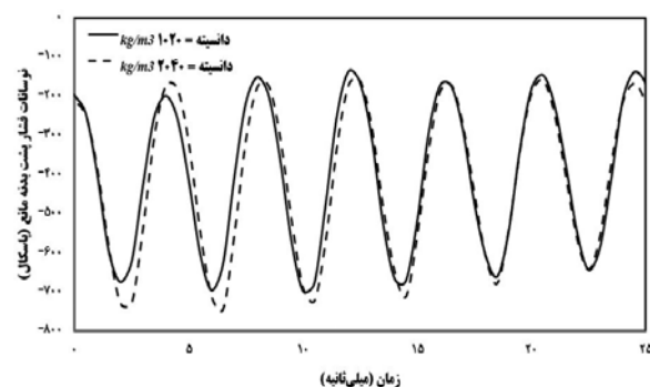
نمودار ۸ اثر چگالی ذرات روی فرکانس گردابه ایجاد شده در پشت بدنه مانع (سرعت ۲۰ m/s، قطر ذرات ۵۰ میکرون و کسر حجمی 10^{-3} )
