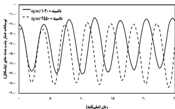
نمودار ۹) تأثیر کسر حجمی ذرات روی فرکانس گردابه ایجادشده در پشت بدنه مانع (سرعت 2.0 \text{ m/s} ، قطر ذرات 50 \text{ }\mu\text{m} و میزان بارگذاری جرمی ذرات 25\% )
