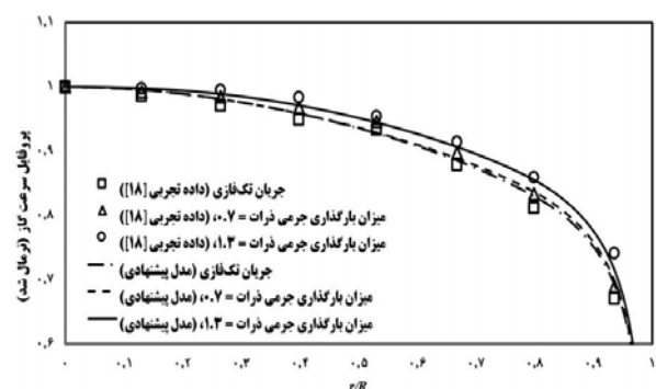
نمودار ۲) مقایسه پروفایل سرعت فاز گاز براساس نتایج به دست آمده از شبیه سازی و داده های تجربی گزارش شده توسط سوچی و همکاران [18] (قطر ذرات ۵۰۰ میکرون)
