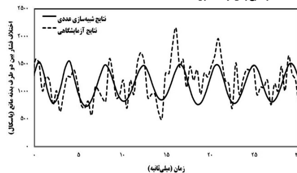
نمودار ۶ مقایسه بین نتایج به‌دست‌آمده از شبیه‌سازی عددی و داده‌های آزمایشگاهی در اندازه‌گیری افت فشار بین دو طرف بدنه مانع در جریان دوفازی گاز-ذره (سرعت ۱۲/۵ m/s، قطر ذرات ۴۰ میکرون، کسر حجمی 10^{-4} و چگالی 2200 \text{ kg/m}^3 )
