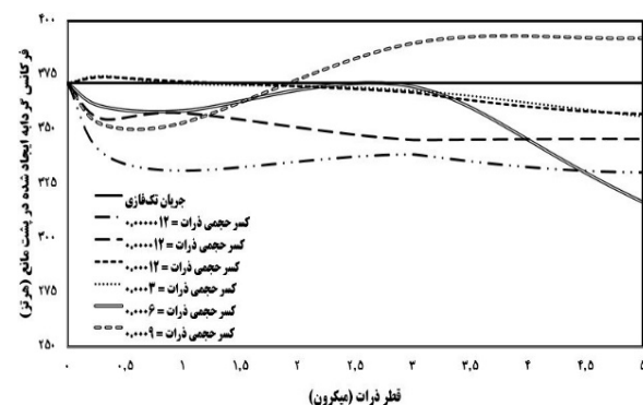
نمودار ۱۱) اثر میکروذرات روی فرکانس گردابه‌های تشکیل‌شده در پشت بدنه مانع در مقادیر مختلف کسر حجمی ذرات (سرعت 2.0 \text{ m/s} و چگالی 1020 \text{ kg/m}^3 )
