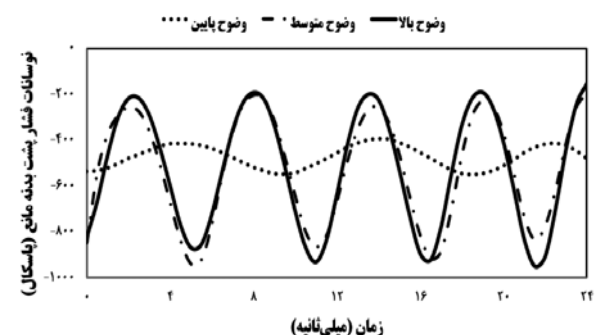
نمودار ۱) توالی زمانی نوسانات فشار (فرکانس گردابه) در پشت بدنه مانع برای اندازه های مختلف از شبکه بندی
