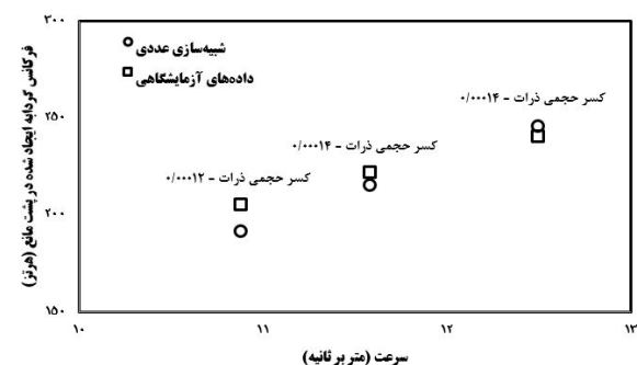
نمودار ۷ مقایسه بین نتایج به‌دست‌آمده از شبیه‌سازی عددی و داده‌های آزمایشگاهی در اندازه‌گیری فرکانس گردابه‌ها در جریان دوفازی گاز-ذره (قطر ذرات ۴۰ میکرون و چگالی ذرات 2200 \text{ kg/m}^3 )
