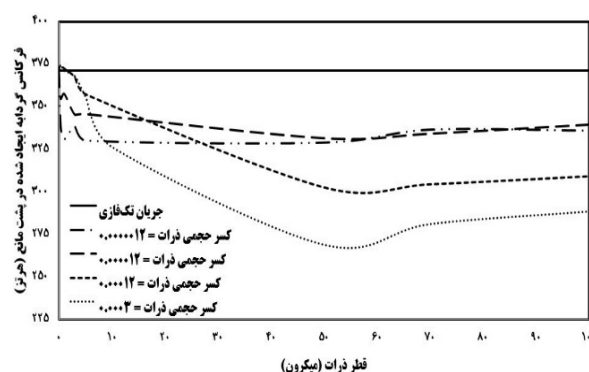
نمودار ۱۰) فرکانس گردابه‌های تشکیل‌شده در پشت بدنه مانع در مقادیر مختلف از کسر حجمی و قطر ذرات (سرعت 2.0 \text{ m/s} و چگالی 1020 \text{ kg/m}^3 )
