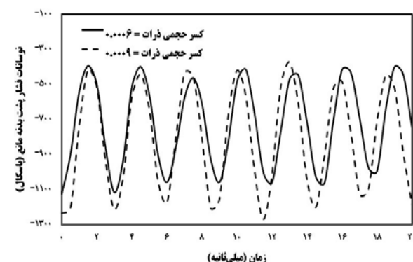
نمودار ۱۲) فرکانس گردابه‌های تشکیل‌شده در پشت بدنه مانع در کسرهای حجمی زیاد از ذرات و در حضور میکروذرات (سرعت 2.0 \text{ m/s} ، قطر ذرات 3 \text{ }\mu\text{m} و چگالی 1020 \text{ kg/m}^3 )
