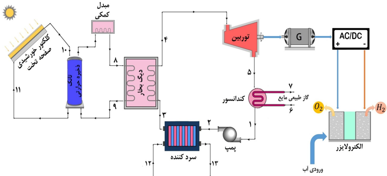
شکل 1 دیاگرام شماتیک سیستم تولید همزمان هیدروژن / سرمایه
