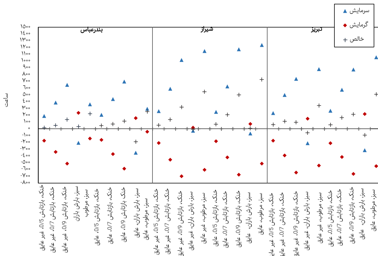
نمودار ۴) کاهش تعداد ساعات سالیانه تهویه مطبوع ساختمان برای سقف‌های مختلف نسبت به سقف معمولی
