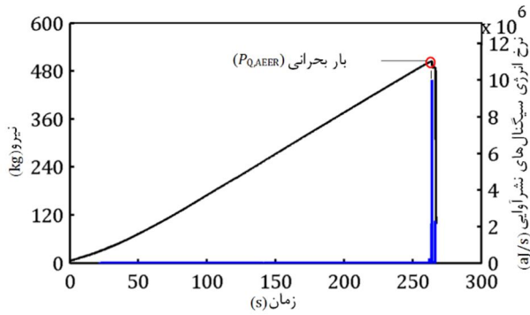
شکل 15 تعیین بار بحرانی به روش نرخ انرژی سیگنال‌های نشر آوابی در نمونه C
