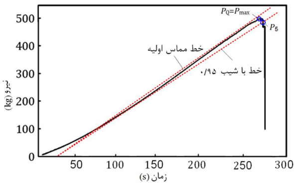
شکل 5 نمودار نیرو-زمان و تعیین بار بحرانی نمونه D
