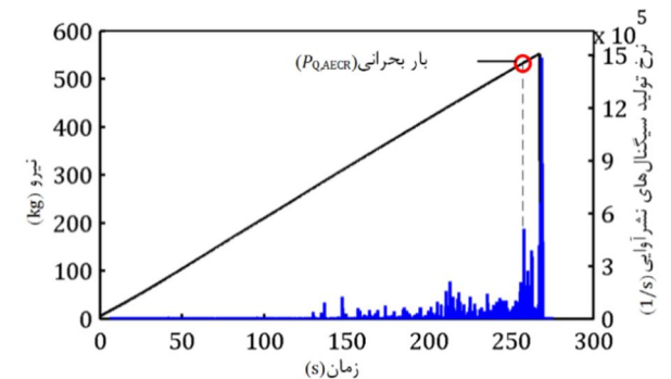
شکل 13 تعیین بار بحرانی به روش نرخ تولید سیگنال‌های نشر آوابی در نمونه E
