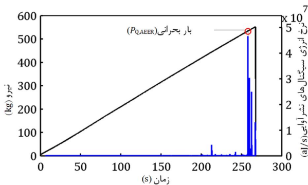
شکل 16 تعیین بار بحرانی به روش نرخ انرژی سیگنال‌های نشر آوابی در نمونه E
