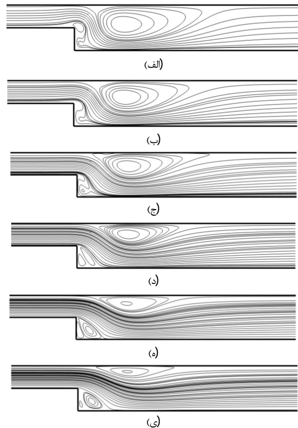
شکل 12 تاثیر عدد رینولدز بر جریان سیال V=18\text{ kV} , \alpha = 45^\circ (الف) \text{Re}=770 (ب) \text{Re}=1050 (ج) \text{Re}=1330 (د) \text{Re}=1610 (ه) \text{Re}=1890 (و) \text{Re}=2170 (ز)
