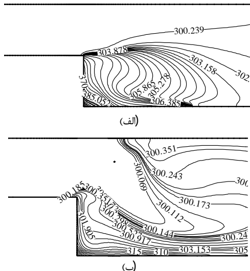
شکل 10 خطوط هم دما ( \alpha = 45^\circ ) الف) V=0 \text{ kV} ب) V=18 \text{ kV}
