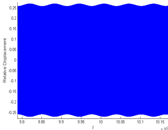
Fig. 12 Time history response diagram of the system for d=0.12 , F=2 and \alpha=0.2 (occurrence of WMR) شکل 12 پاسخ زمانی سیستم به ازای \sigma=2 , d=0.12 , F=2 , \alpha=0.2 (رخداد پاسخ مدوله ضعیف)
