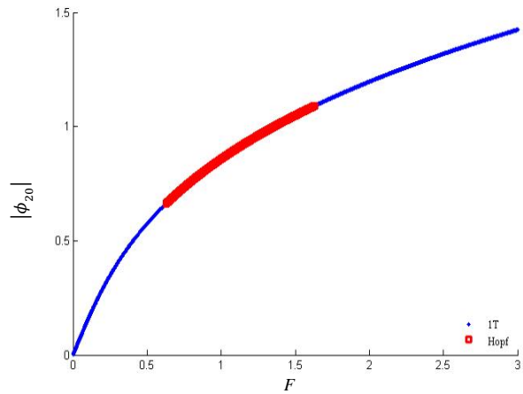
Fig. 13 The Force-response diagram of the system for d=0.5 , \sigma=1 and \alpha=0.2 شکل 13 نمودار پاسخ ماندگار سیستم به ازای تغییرات دامنه تحریک خارجی (1. =) (\alpha d=0.5, \alpha=0.2)
