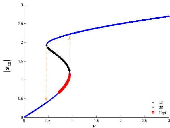
Fig. 14 The Force-response diagram of the system for d=0.24 , \sigma=1 and \alpha=0.2 شکل 14 نمودار پاسخ ماندگار سیستم به ازای تغییرات دامنه تحریک خارجی (1. =) (\sigma d=0.24, \alpha=0.2)
