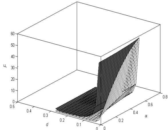
Fig. 2 The existence of the saddle-node bifurcations in the non-dimensional parameter space of F , \alpha and d for \sigma=1 شکل 2 رخداد انشعاب زین اسبی در فضای بی‌بعد پارامتری d (فاصله جاذب از تکیه‌گاه)، F (دامنه تحریک خارجی) و \alpha (دمپینگ جاذب) به ازای \sigma=1
