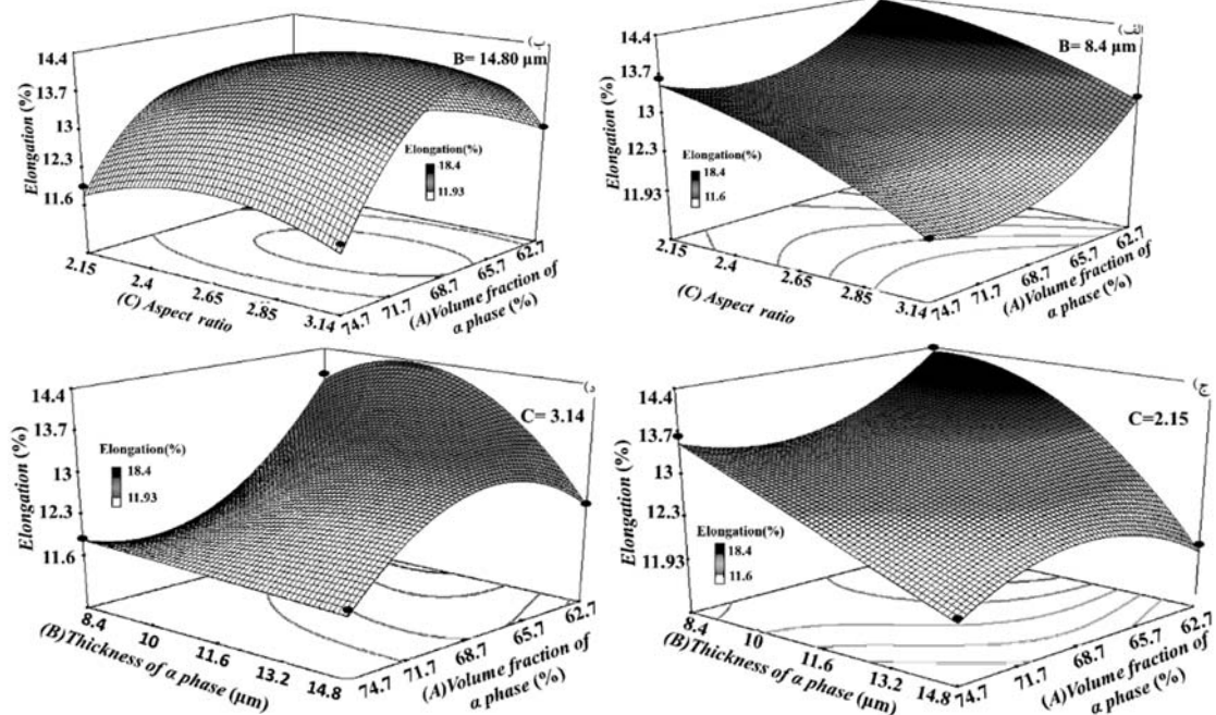
نمودار ۶) رویه پاسخ ازدیاد طول به‌ازای پارامترهای ورودی
