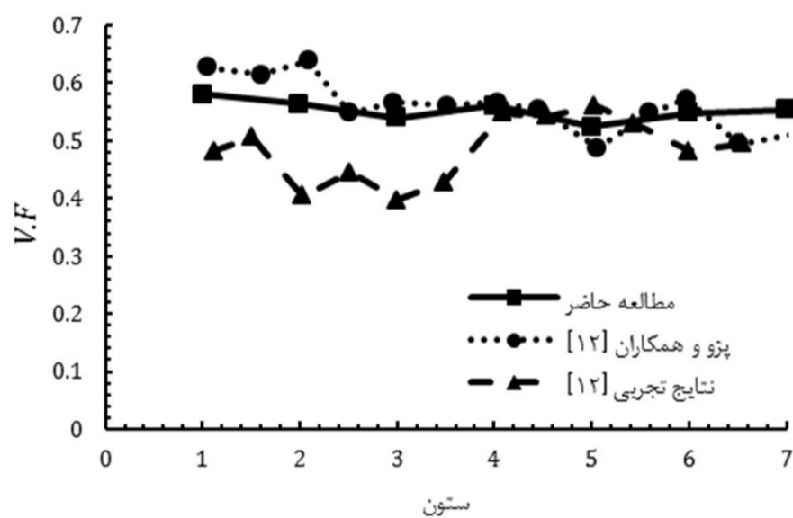
شکل 18 کسر حجمی بخار شار حرارتی 30\text{kW/m}^2 در فاصله بین ردیف 13 و 14
