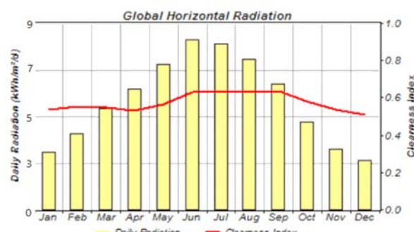
نمودار (۲) منحنی میانگین ماهانه تابش افقی برای ۱۰ سال در شهرستان میانه رفرنس میانه
