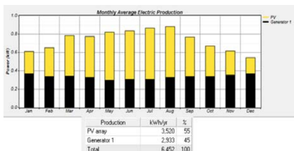
نمودار ۱۱) نتایج مربوط به میانگین تولید برق ماهیانه در آرایش دیزل-فوتوولتائیک
