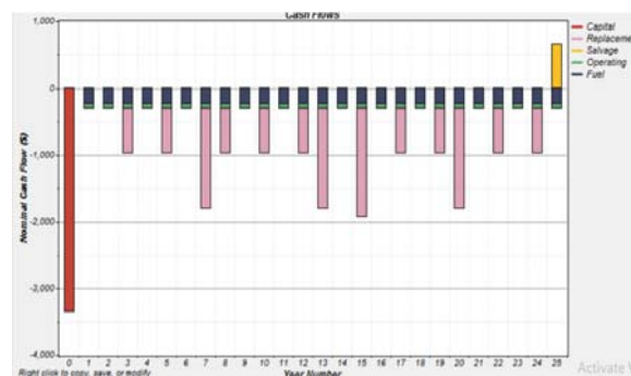
نمودار ۱۰) شرح روند موجودی در چرخه عمر برای آرایش تک‌گانه ژنراتور دیزلی
