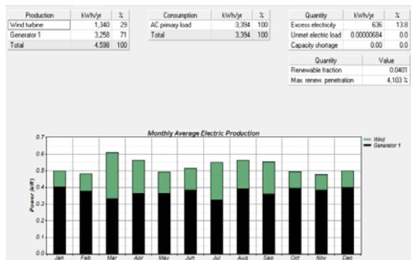
نمودار ۲۲) نتایج مربوط به میانگین تولید برق ماهیانه در آرایش ژنراتور دیزل- توربین بادی در ارتفاع ۳۰ متری
