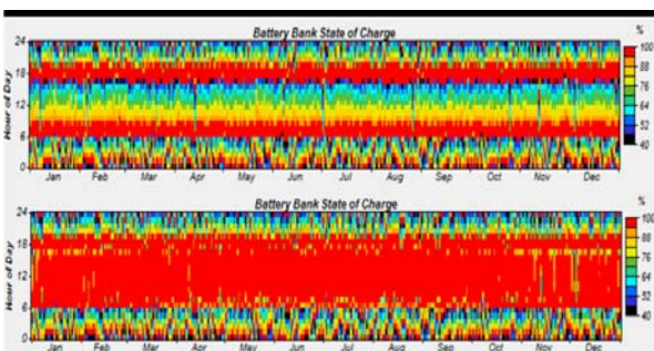
نمودار ۱۲) پروفیل مقایسه مربوط به وضعیت شارژ و دشارژ باتری‌ها، آرایش تکی ژنراتور دیزلی (بالا)، آرایش ژنراتور به همراه آرایه فوتوولتائیک (پایین)
