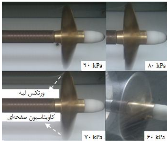
شکل ۱۱ مراحل شروع و توسعه کاویتاسیون در تونل کاویتاسیون با افت فشار در محدوده ۹۰-۶۰ kPa در J=0.2
