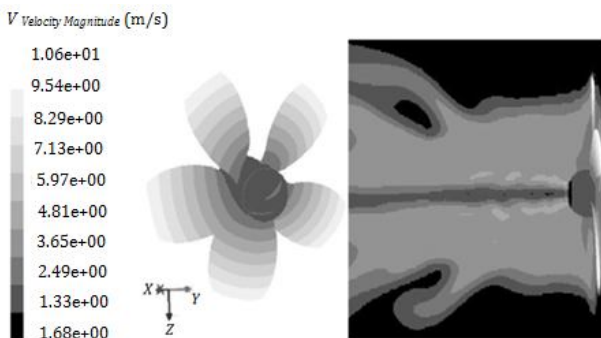
شکل ۷- ب کانتور میدان سرعت جهت محاسبه عدد کایتاسیون در J=0.12
