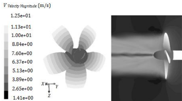
شکل ۸- ب کانتور میدان سرعت جهت محاسبه عدد کاپیتاسیون در ۰/۱۷ J=
