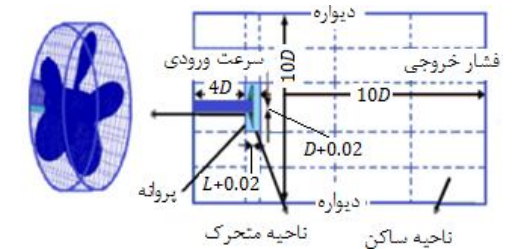
شکل ۳ شبکه‌بندی پروانه، ناحیه محاسباتی حل و اعمال شرایط مرزی
