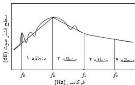
شکل ۲ محدوده فرکانسی نویز پروانه در حالت کاویتاسیونی [۴]
